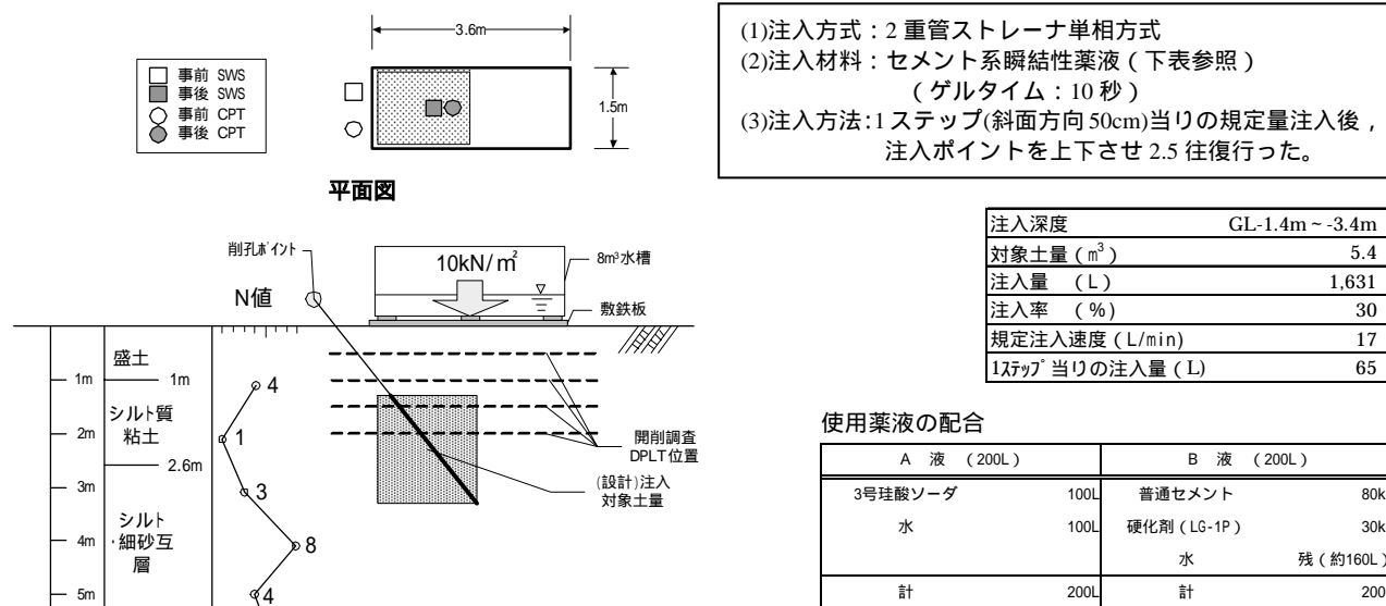
図1 試験位置図と注入条件
