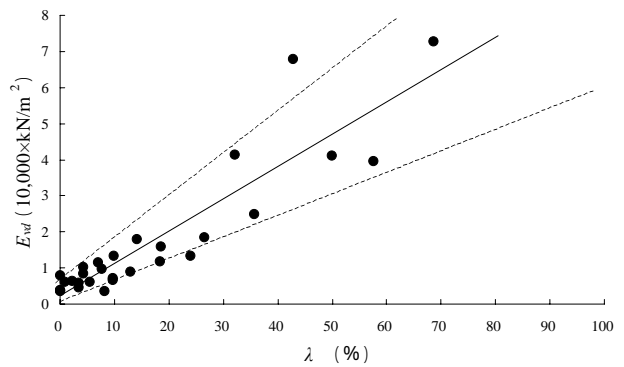
図4 と E_{vd} の関係(DPLT)
