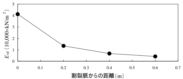
図5 割裂脈からの水平距離と E_{vd} の関係(DPLT)
